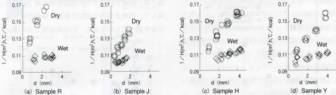
図4 Estimation of H values
